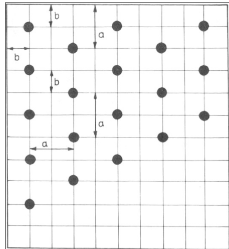
A fólialyukasztás vázlata különböző lyukbősségnél 200 lyuk/m 2 : a = 7,1 cm, b = 3,5 cm 400 lyuk/m 2 : a = 5,0 cm, b = 2,5 cm 600 lyuk/m 2 : a = 4,1 cm, b = 2,0 cm 800 lyuk/m 2 : a = 3,5 cm, b = 1,8 cm 1000 lyuk/m 2 : a = 3,2 cm, b = 1,6 cm
